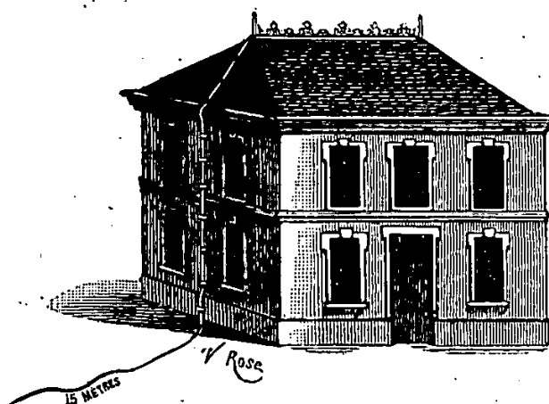
Fig. 47. Maison pourvue du circuit des faites et ne portant que des pointes de hauteur médiocre, juste suffisantes pour déterminer la marche du fluide. Dans ce cas le peril-fluide peut être placé dans la terre végétale.
