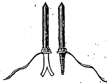
Fig. 49. Tiges du paratonnerre pour tous portant leurs modes d'attacho et leurs rubans en cuivre.
