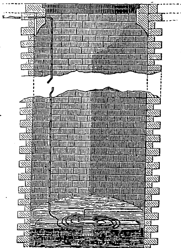
Fig. 23. Perd-fluide roulé en spirale placé dans le fond d'un puits.
