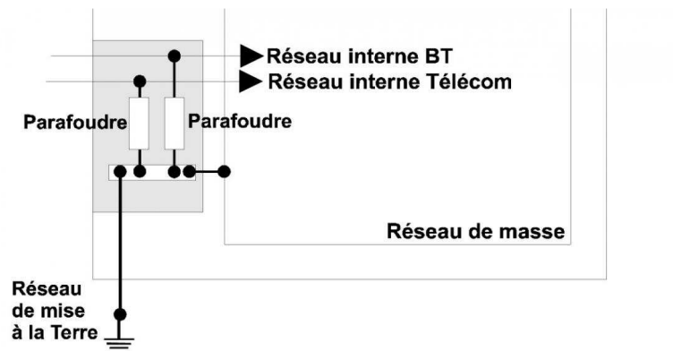
Schéma de mise en œuvre optimisée des Parafoudres BT et Télécommunications
